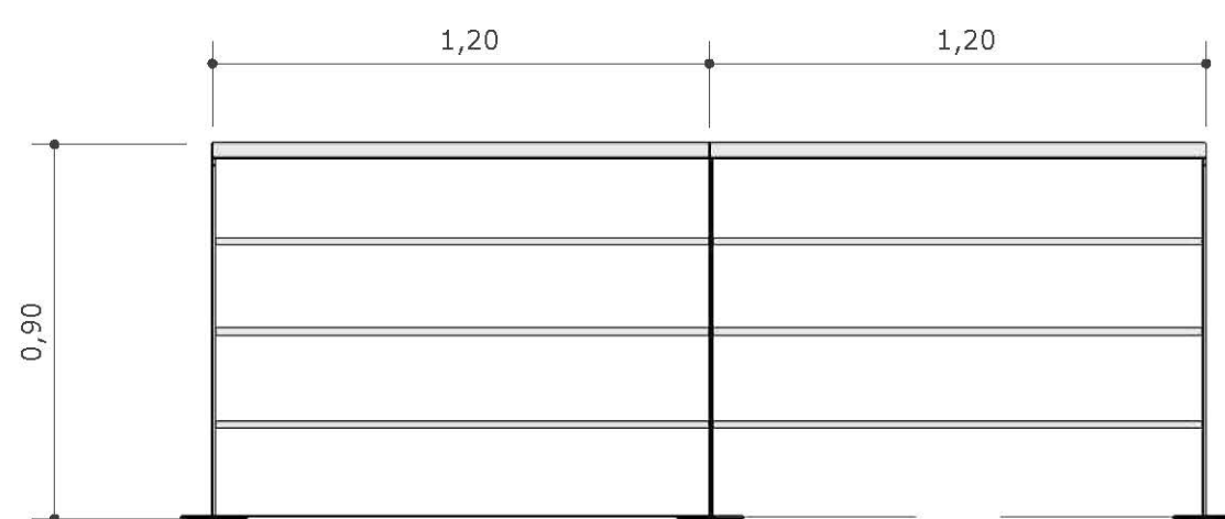
DETTAGLIO PROSPETTO PASSAMANO
