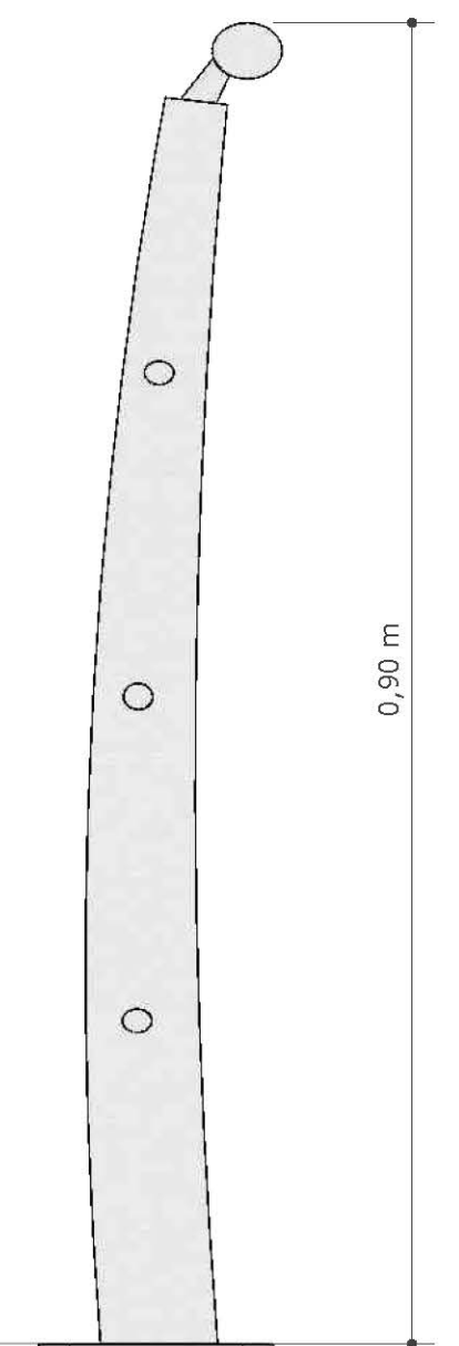
DETTAGLIO PROFILO PASSAMANO
