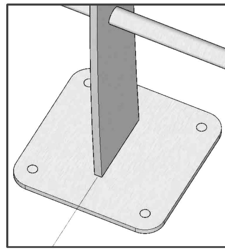
DETTAGLIO PIASTRA ANCORAGGIO
